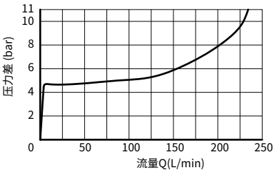
GWEH25.../6B2... 型
