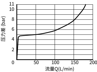
GWEH16.../6B2... 型
