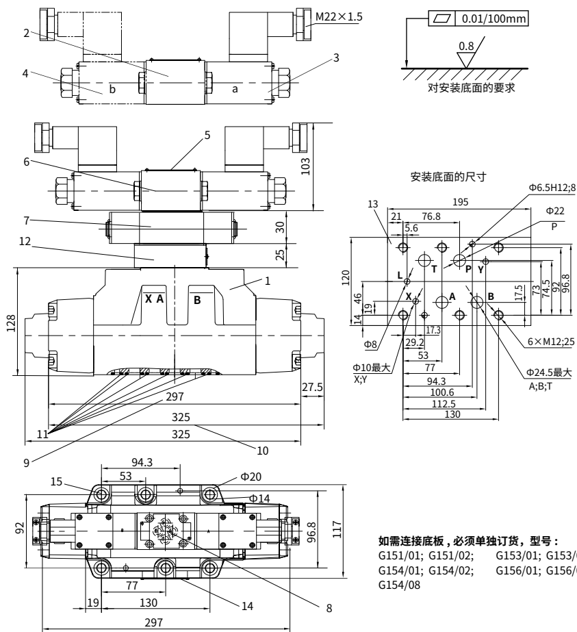
GWEH25../6B2.. 型电液换向阀外形尺寸图
