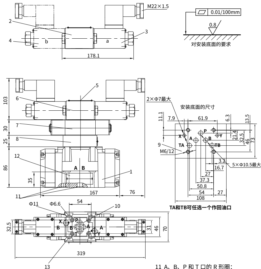
GWEH10../6B2.. 型隔爆电液换向阀外形尺寸图
