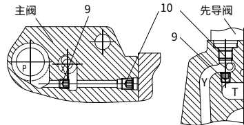
GWEH16.../6B2...型供排结构图
